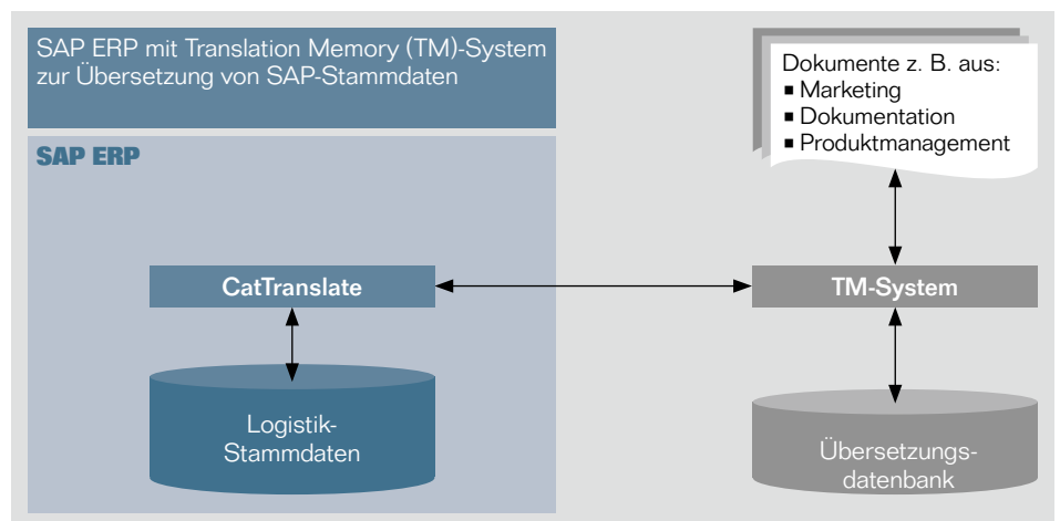
Abb. 3: Prozesssicht zum Anschluss von SAP ERP an Translation-Memory-Systeme
